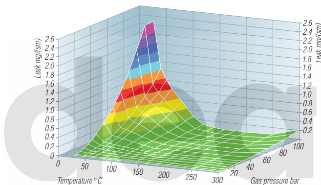
Gasket load 15 MPa
